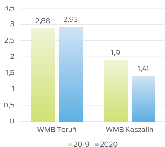
Wykres nr 2. Porównanie całkowitej emisji zanieczyszczeń do powietrza do czasu pracy wytwórni mas bitumicznych w latach 2019-2020 [Mg]
