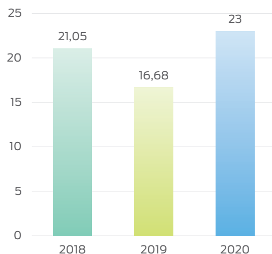
Wykres nr 8. Zbiorcze zestawienie poziomu emisji CO dla WMB Toruń w latach 2018-2020 [Mg]
