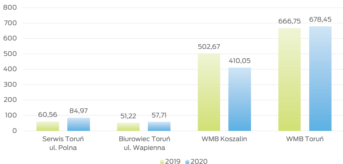
Wykres nr 23. Porównanie poziomu zużycia energii elektrycznej w okresie 2019-2020 [MWh] w jednostkach stacjonarnych
