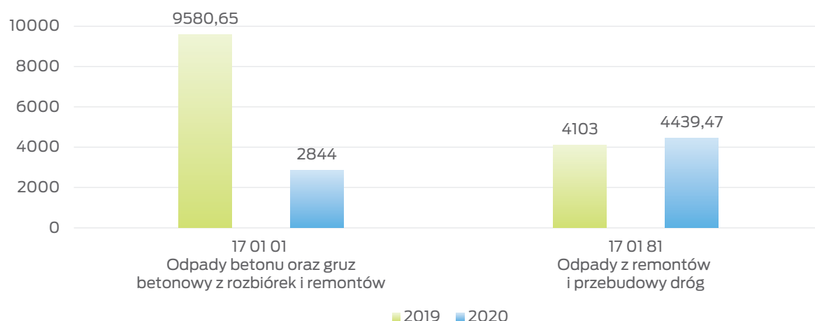
Wykres nr 29. Rodzaje i ilość odpadów poddana odzyskowi w WMB Toruń w latach 2019-2020 [Mg]
