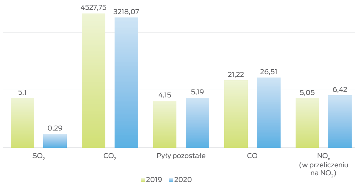
Wykres nr 3. Zbiorcze zestawienie zanieczyszczeń wyemitowanych przez WMB w okresie 2019-2020 [Mg]
