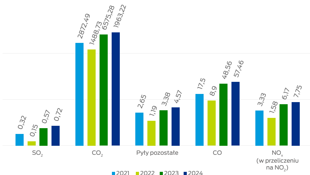
Wykres nr 3. Zbiorcze zestawienie zanieczyszczeń wyemitowanych przez WMB w okresie 2021-2024 [Mg]
