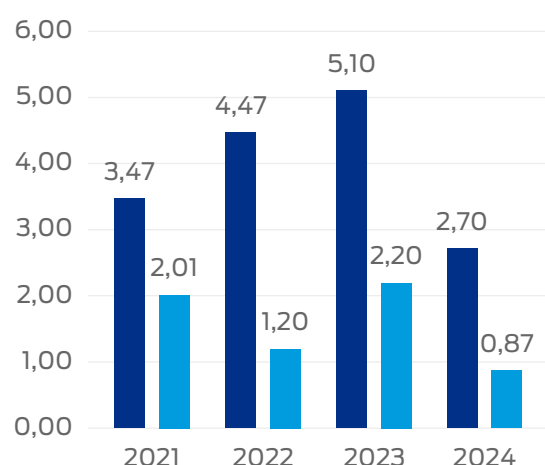
Wykres nr 2. Porównanie catkowej emisji zanieczyszczeń do powietrza do czasu pracy wytwórni mas bitumicznych w latach 2021-2024 [Mg]
